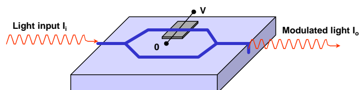
Mach-Zehnder interferometer
